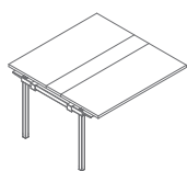
SY52 1200 / 1210 / 740 48.2 kg
