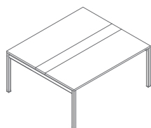
SY26 1600 / 1410 / 740 75.9 kg
