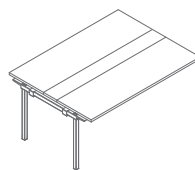
SY56 1600 / 1210 / 740 62.1 kg
