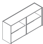
V27 1628 / 424 / 807 79 kg
